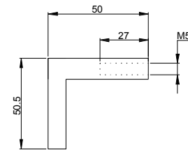
DS Fixing Bolt 2PCS
