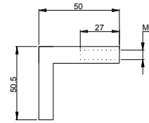
DS Fixing Bolt 2PCS
